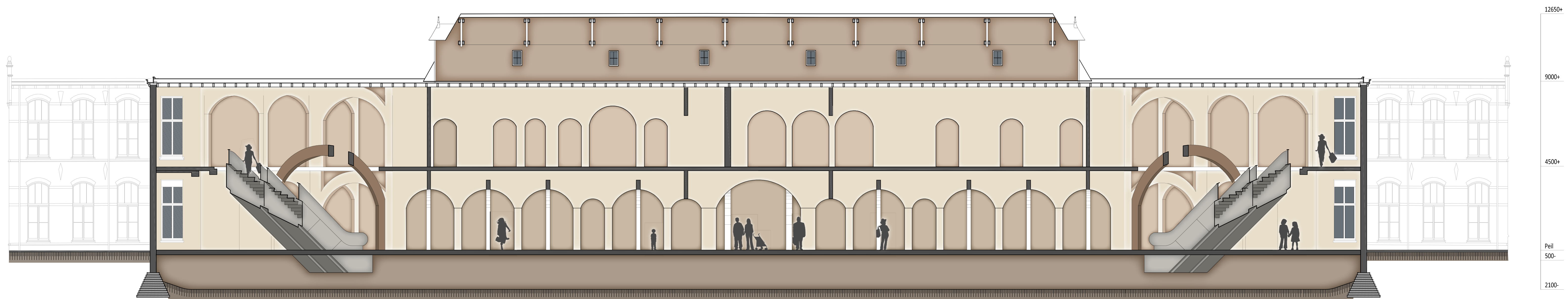
Doorsnede CC'
