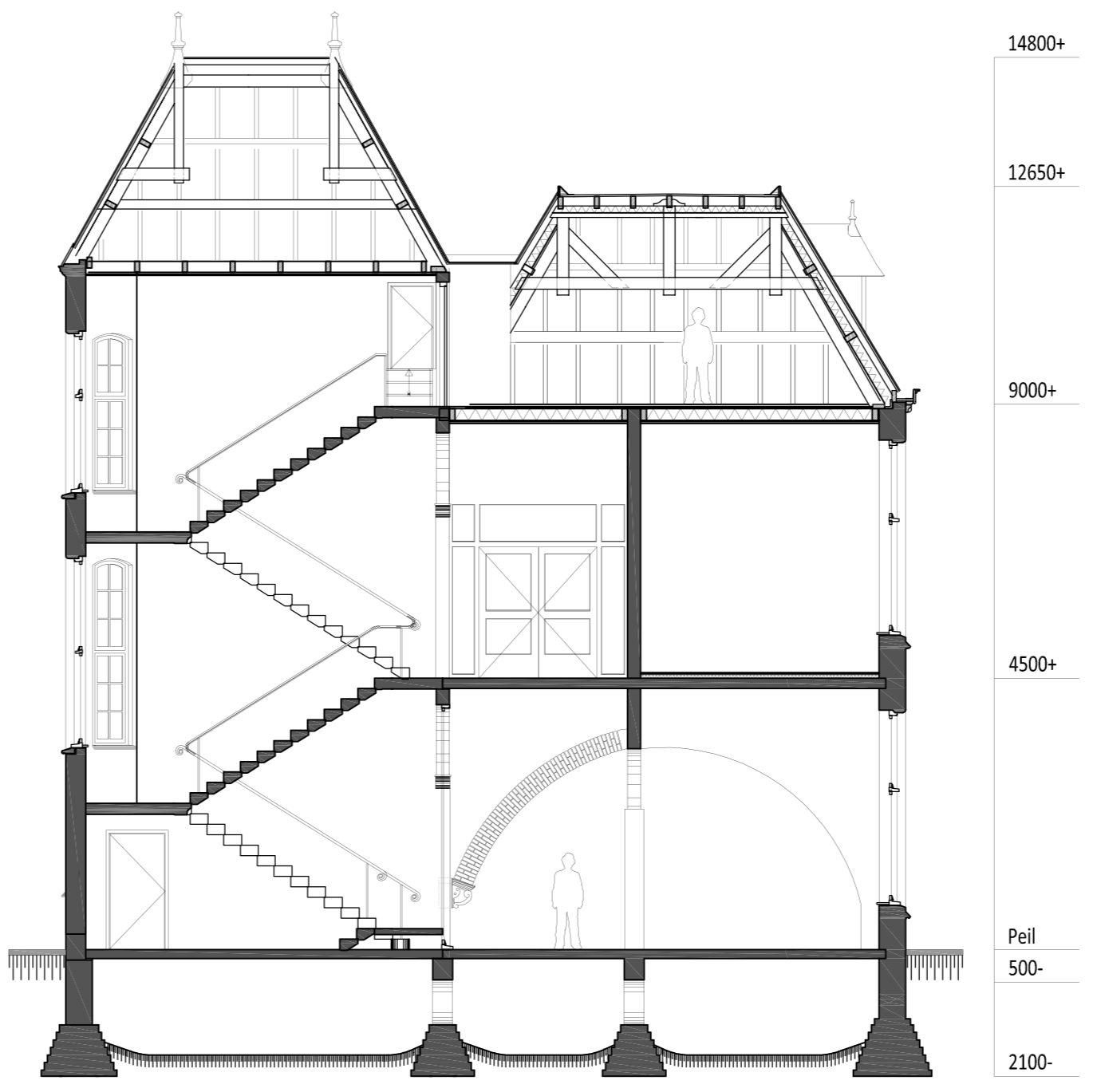
Doorsnede BB'
